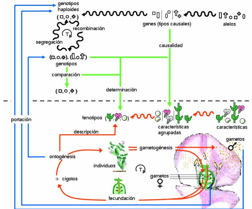
Figura 2: Grafo conceptual de la Genética Mendeliana
